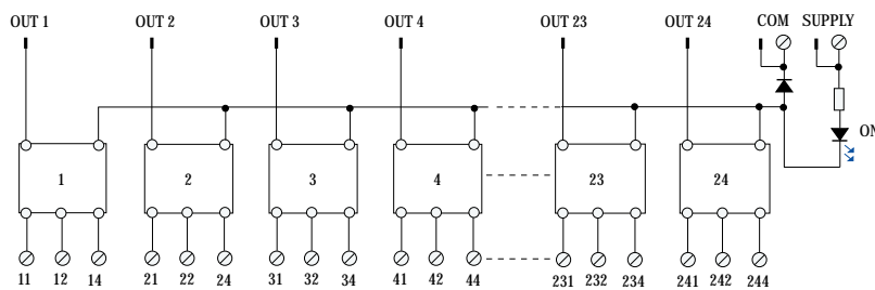
SCHEMA A BLOCCHI MODULO 24 USCITE 24 OUTPUT MODULE BLOCK DIAGRAMS
